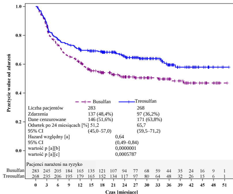
Rycina 1. Estymacja Kaplana-Meiera przeżycia wolnego od zdarzeń (pełna analiza).
